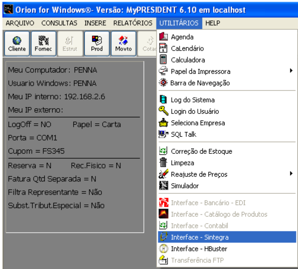
Figura 1 - Interface - Sintegra
