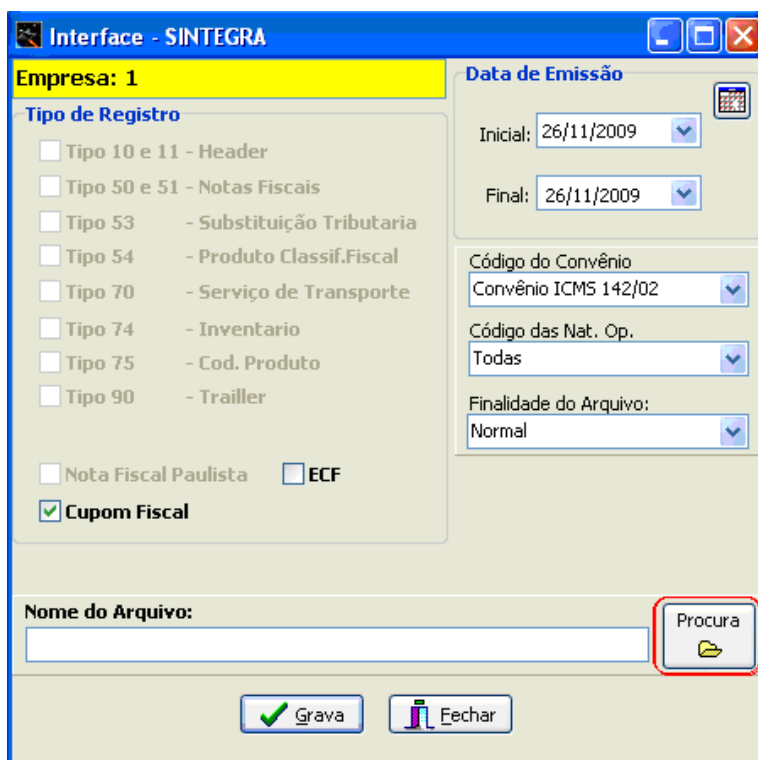
Figura 4 - Selecionando Destino
